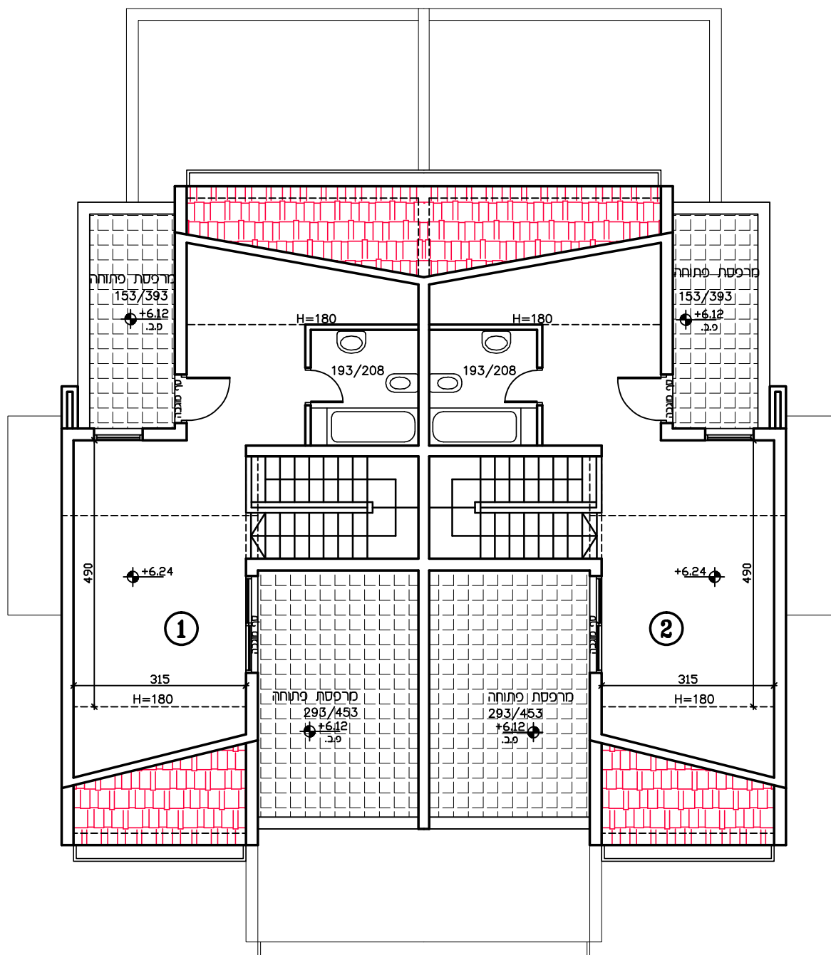
טיפוס A3 תכנית קומה ב' ק.מ. 1:100
