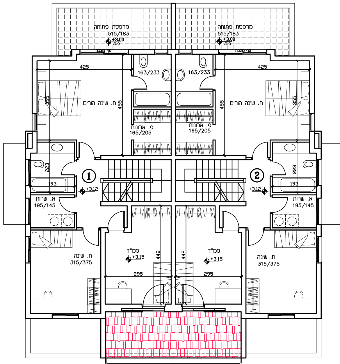
טיפוס A4 תכנית קומה א' ק.מ. 1:100
