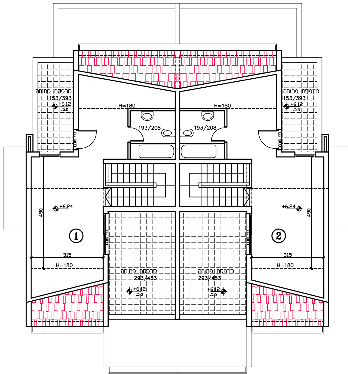
טיפוס A4 תכנית קומה ב' ק.מ. 1:100
